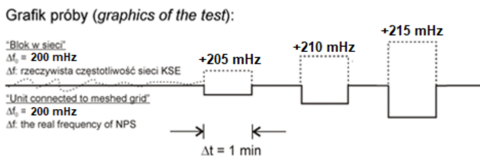
Rys. 1 Sprawdzenie niewrażliwości odpowiedzi częstotliwościowej.
