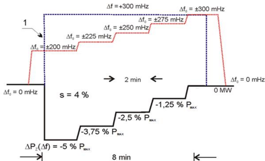
Rys. 4 Sprawdzenie odpowiedzi częstotliwościowej przy zmianach: strefy nieczułości odpowiedź częstotliwościowej, statyzmu oraz odchyłki częstotliwości
