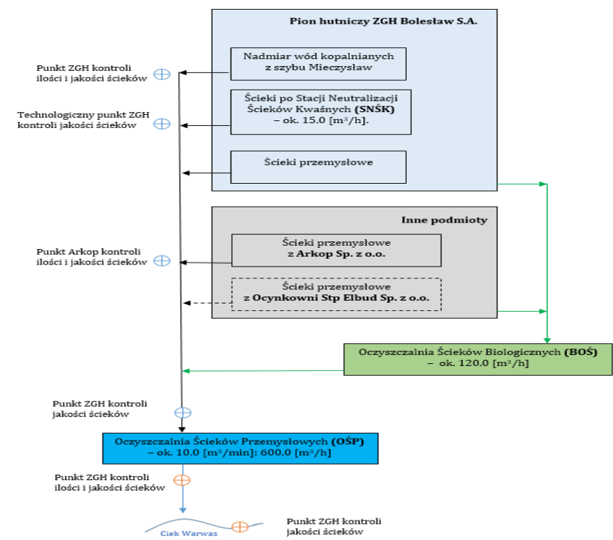
Schemat nr 5. Gospodarka ściekowa rejonu „Bolesław”.
