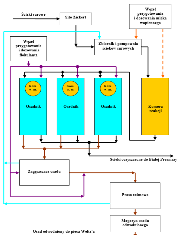
Schemat nr 6. Schemat ideowy oczyszczalni ścieków przemysłowych (OŚP).
